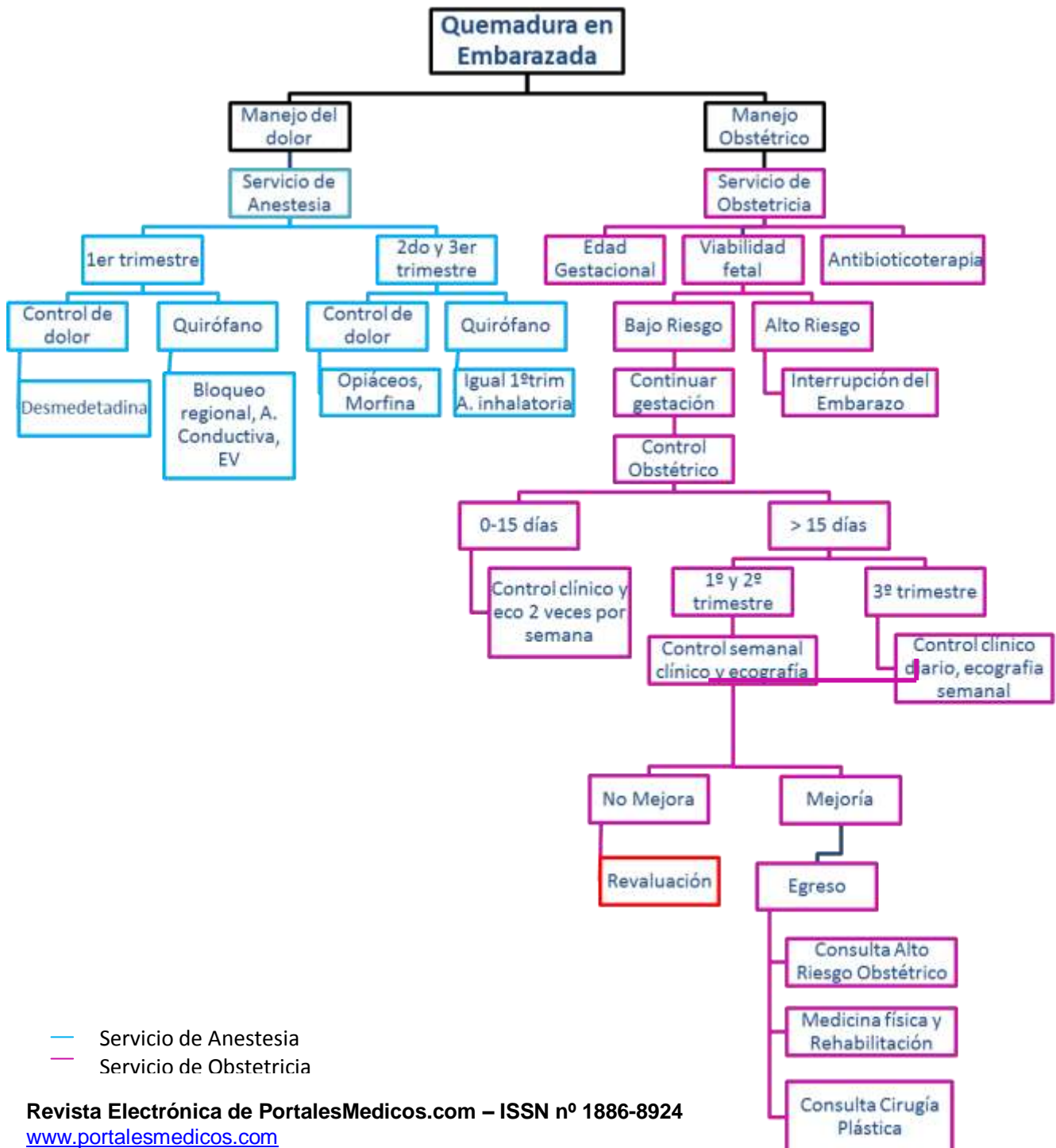
Algoritmo B
